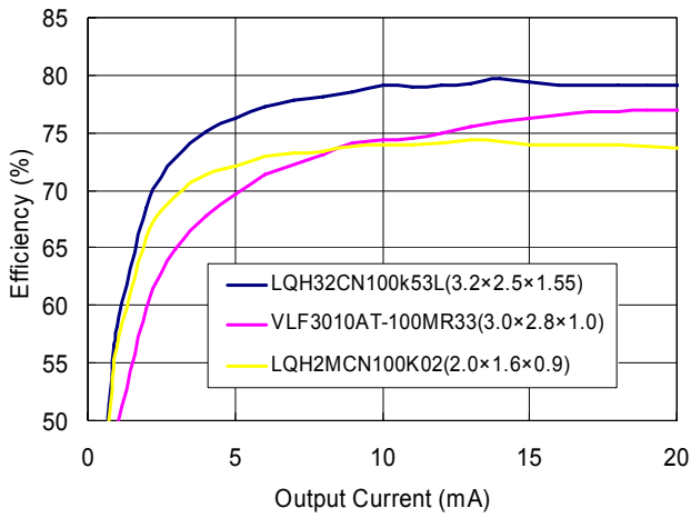
V_{OUT}=20V, V_{IN}=3.6V
